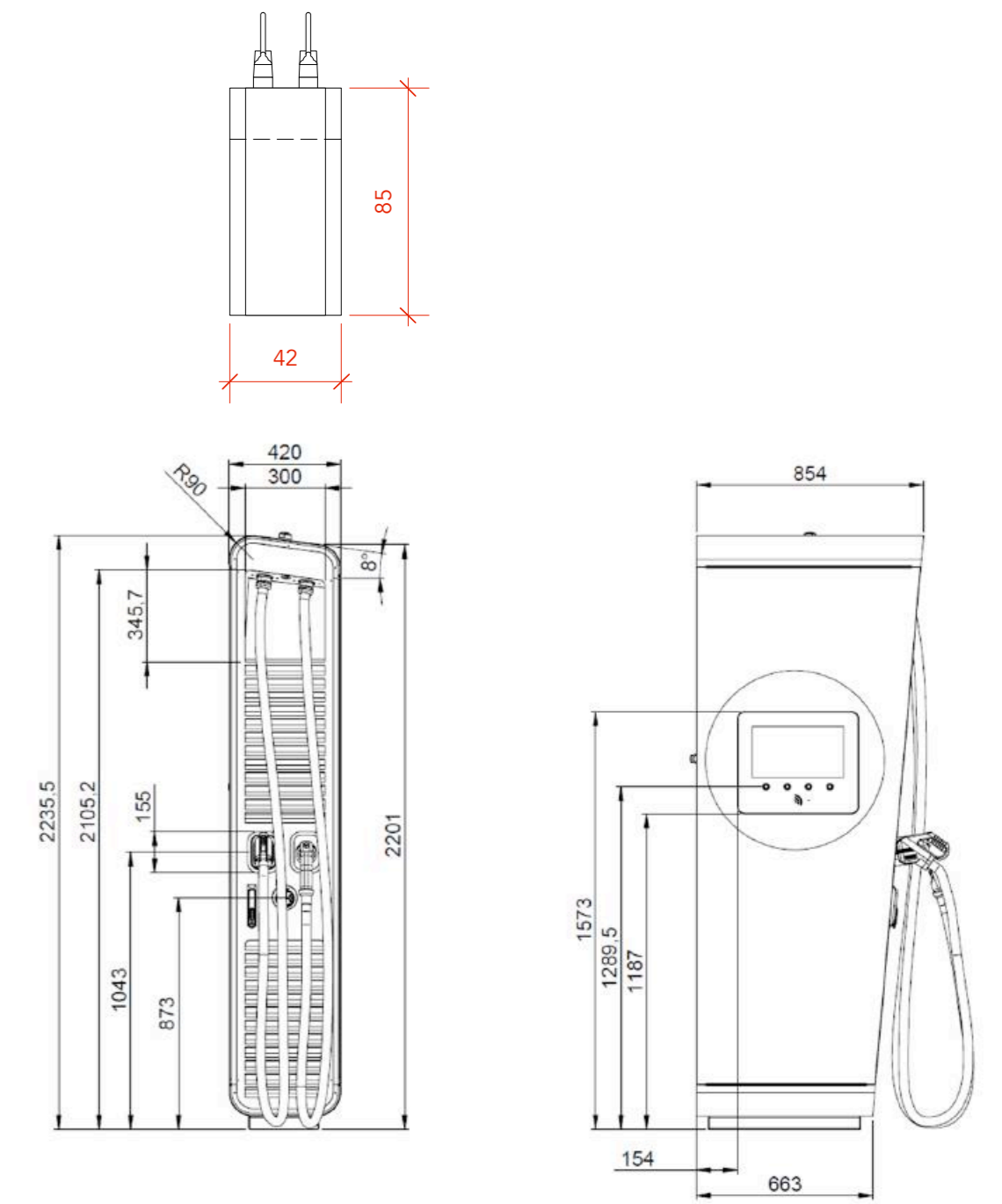
BORNE DE RECHARGE ÉLECTRIQUE 150KW - NON SOUMIS À PERMIS
