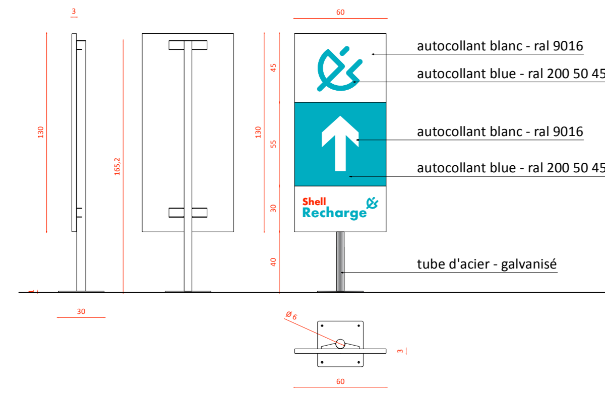
panneau de signalisation de station de chargement
