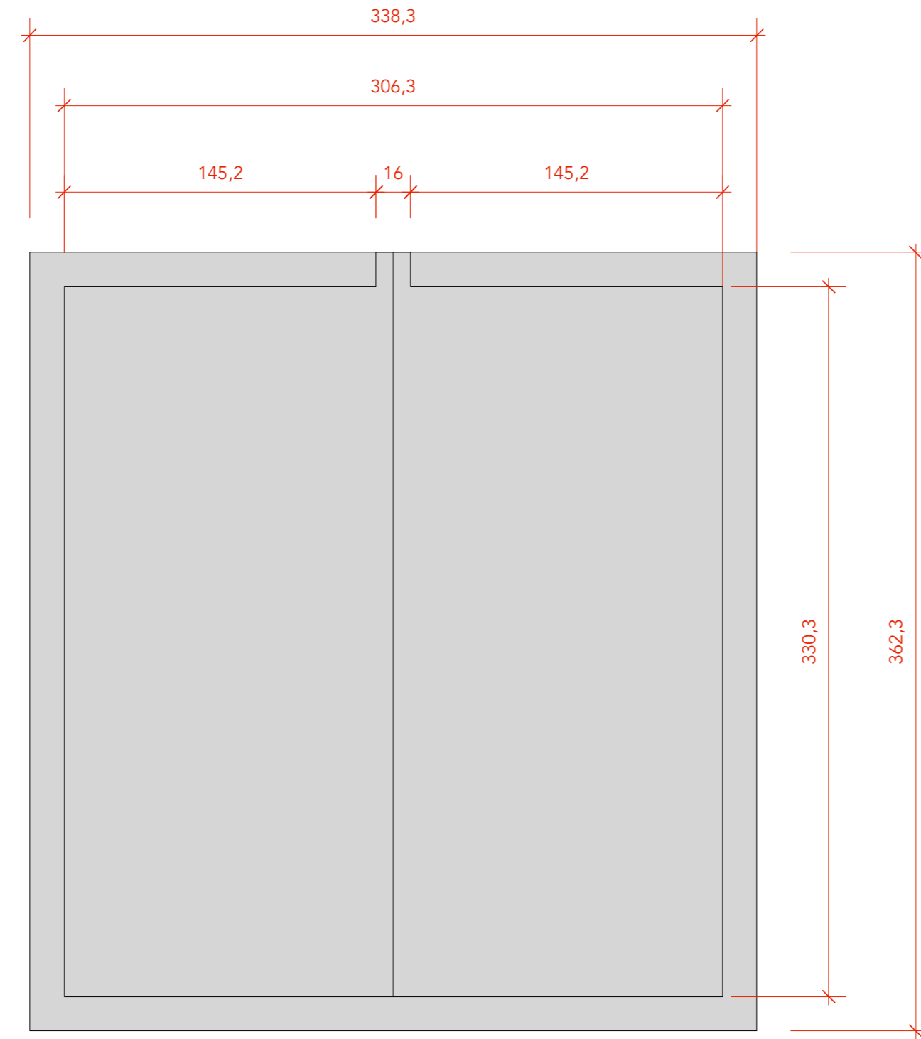
PLAN DU TOIT
