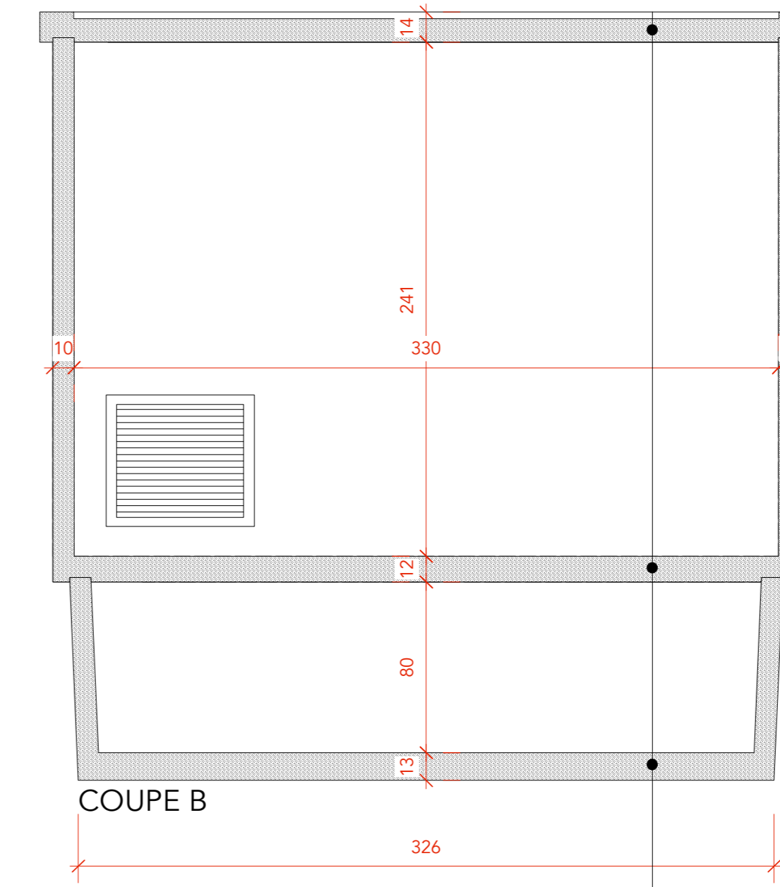
STRUCTURE EN BÉTON ARMÉ
